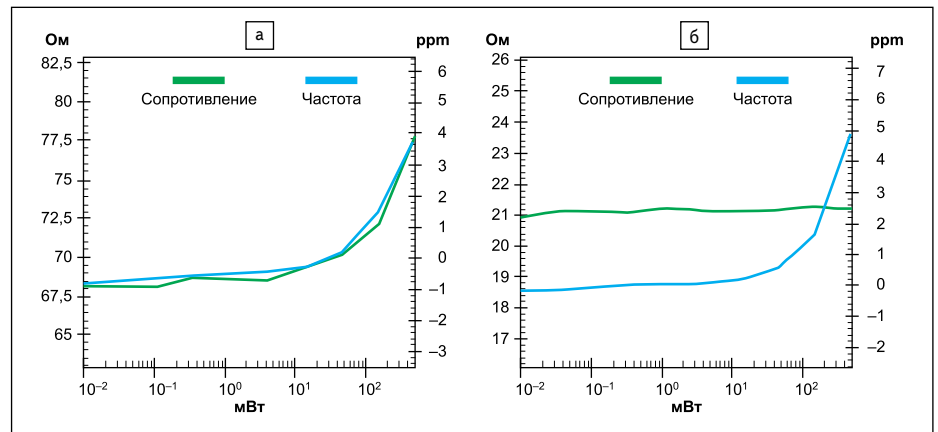
Рис. 3. Зависимость резонансной частоты и динамического сопротивления от уровня возбуждения кристалла
