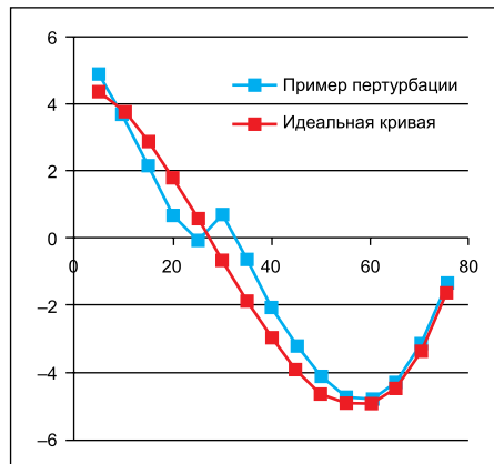
Рис. 4. Температурно-частотная характеристика кварца
