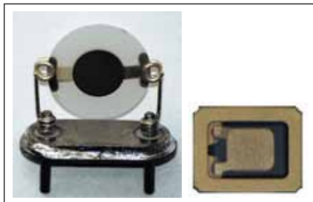
Рис. 2. Сравнение конструкции резонаторов Golledge типа HC49 и GSX-213
